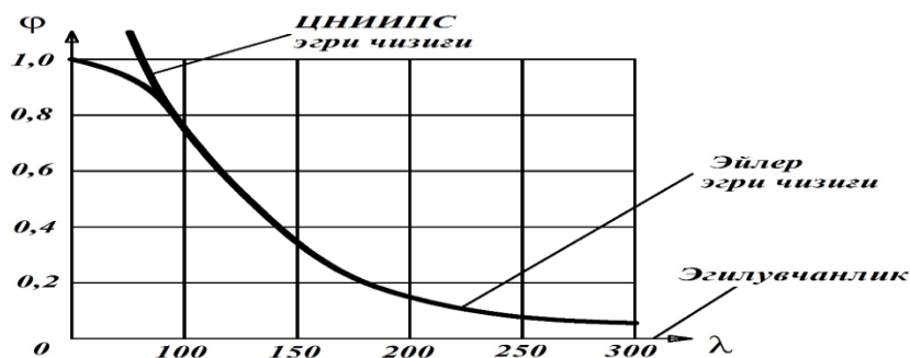
3-rasm. Bo‘ylama egilish koeffisienti va egiluvchanlik diagrammasi.
