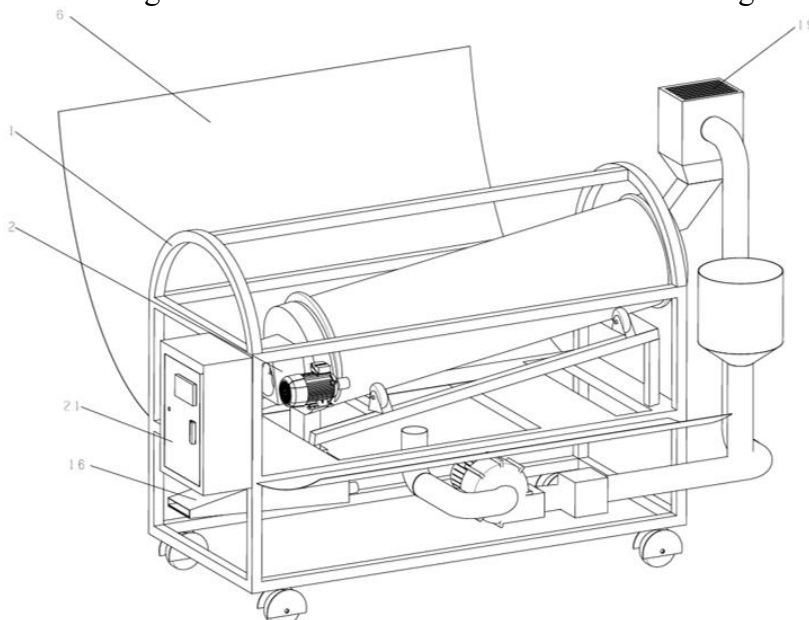
1-rasm. Takomillashtirilgan barabanli don quritgich sxemasi.
