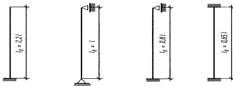
1-rasm. Markaziy siqiluvchi sterjenlarning hisobiy sxemasi.
