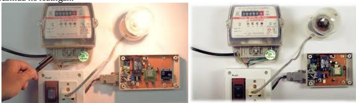
2-rasm. Elektr energiyasini monitoring qilish tizimining prototipi
