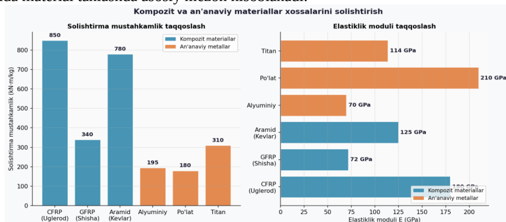
1-diagramma. Kompozit va an'anaviy materiallarning solishtirma mustahkamligi va elastiklik moduli taqqoslash
