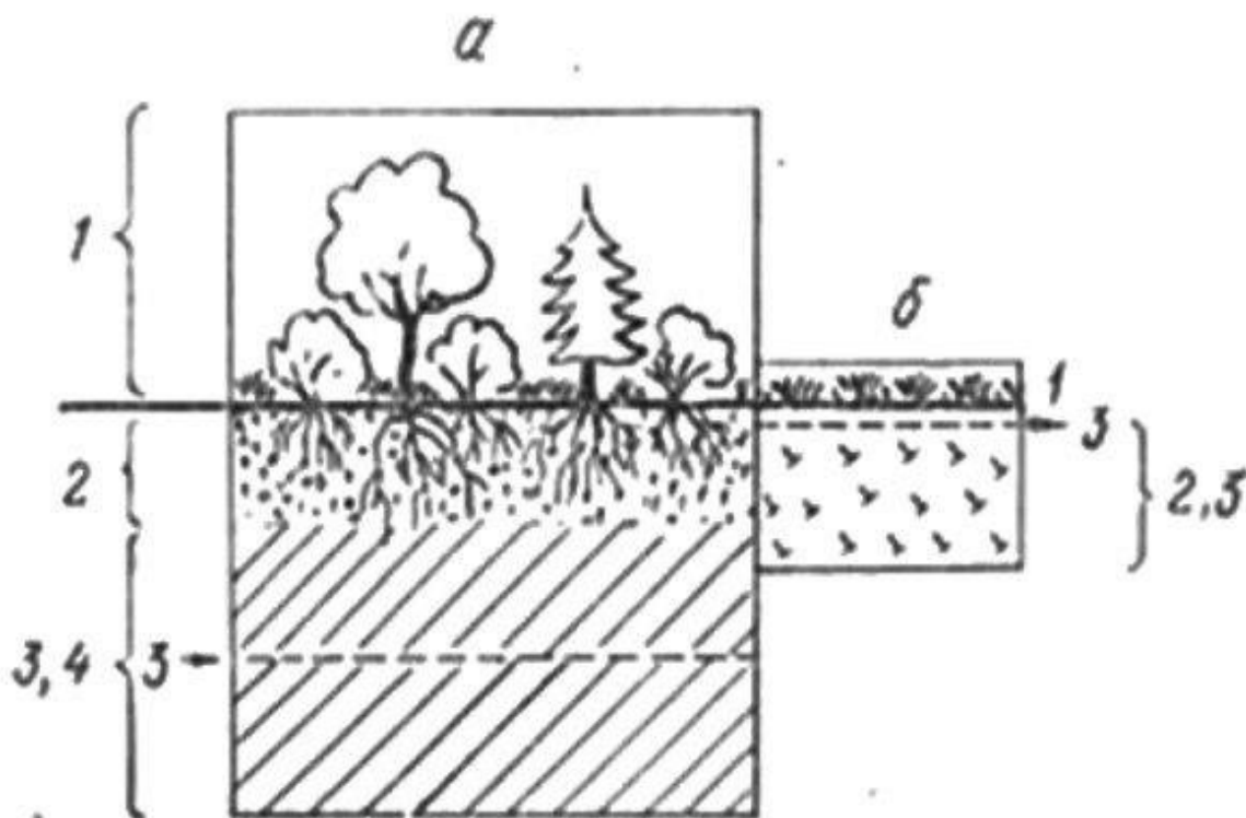
1 – расм. O‘rmon (a) va botqoqlik (b) landshaftlarining vertikal tuzilishi: 1 - tirik modda qatlami, 2 - tuproq, 3 - yer osti suvlari, 4 - nurash qobig‘i
