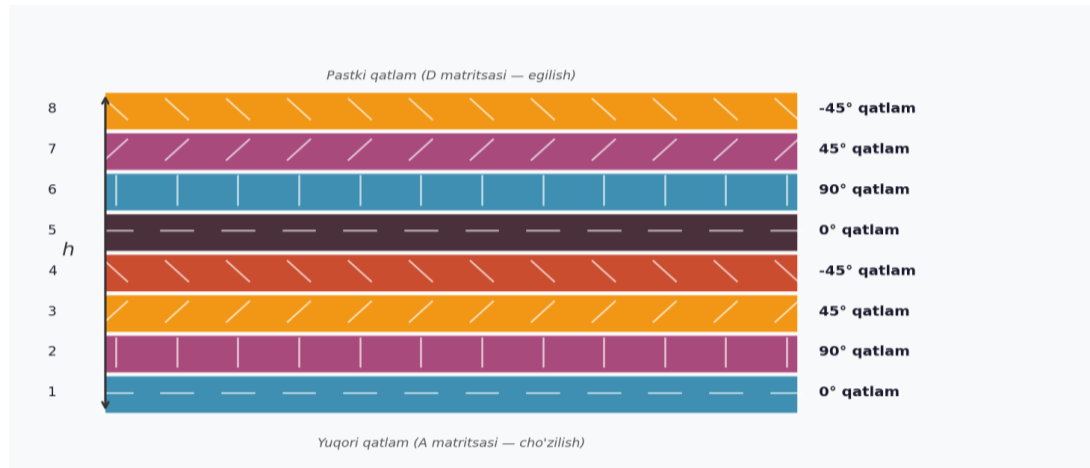
1-rasm. Kompozit laminat plastinkaning qatlam tuzilishi va A-B-D matritsasi komponentlari
