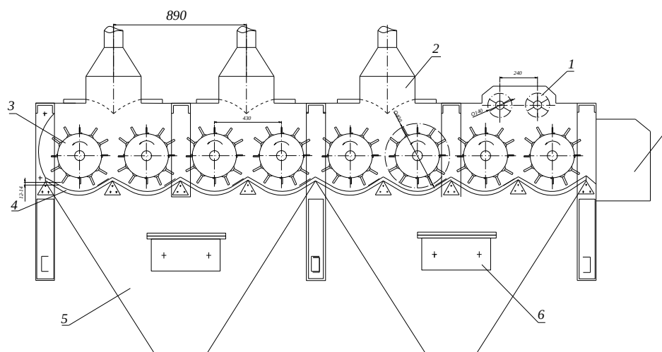
2-rasm. Taklif etilayotgan quritish tozalash jarayonlari mavjud bo‘lgan 1XK uskunasi-ning ko‘ngdalang qirqim sxemasi
